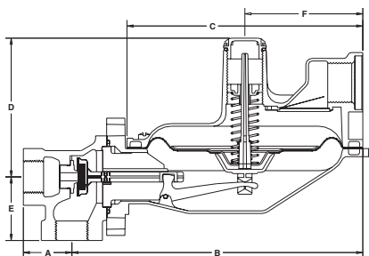
1813C - 90°
