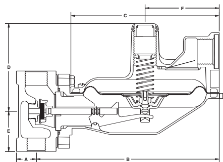
1803B2 - 180°
