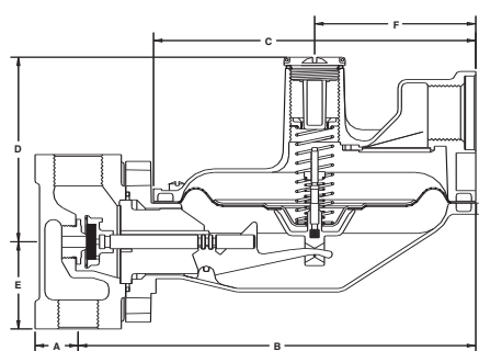
1813B2 - 180°
