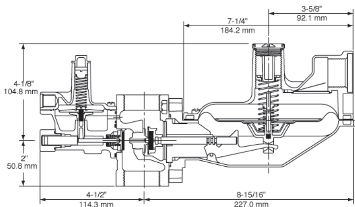
1843B2-HC
