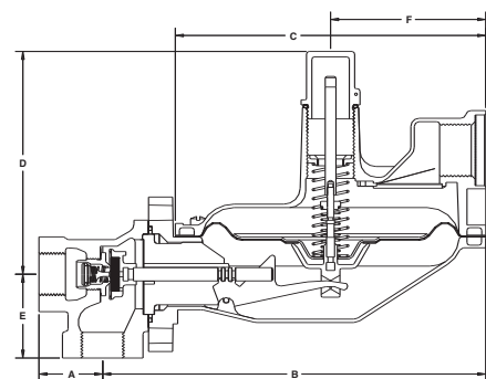
1833B2 - 90°
